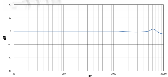
i436 – Zertifiziertes Messmikrofon nach IEC 61672 Class 2
